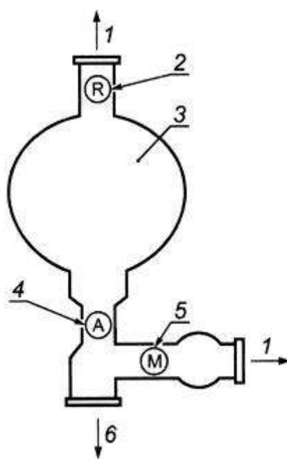
Рисунок F.5 - Схема пипетки
