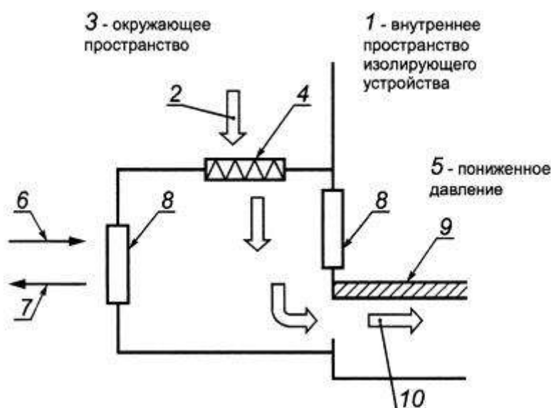
Рисунок D.6 - Передаточное устройство типа C2
