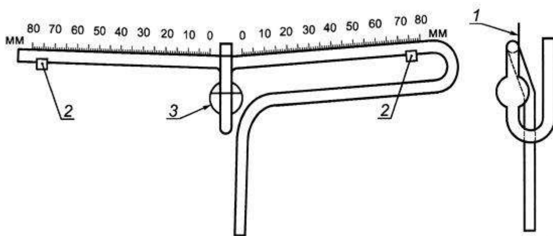
Рисунок F.4 - Трубка Парджо (тип А)
