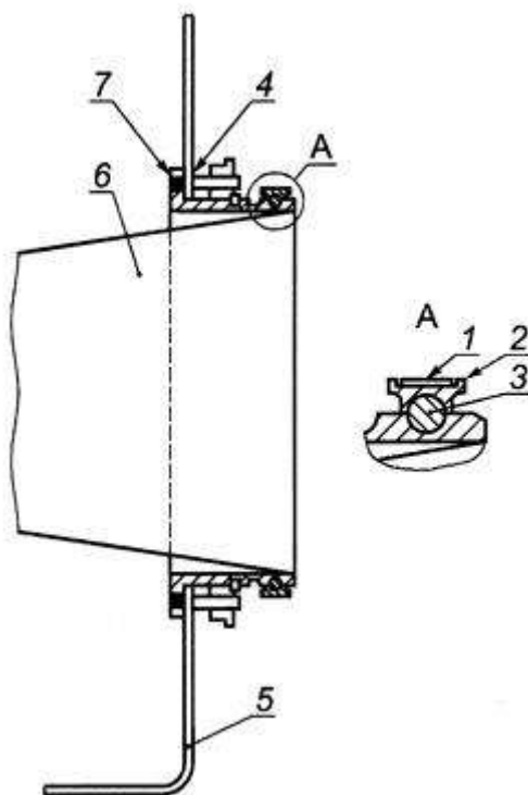
Рисунок С.1 - Перчаточный порт и перчаточный узел
