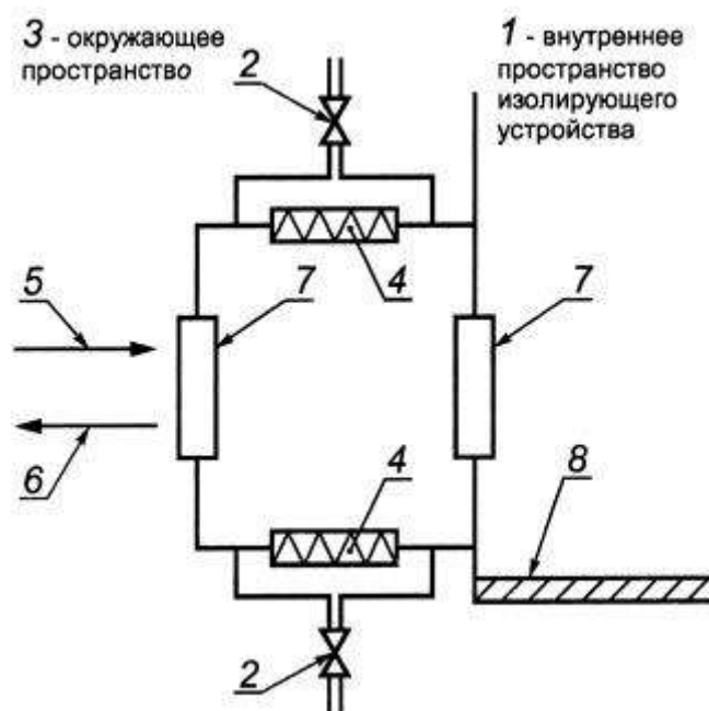
Рисунок D.7 - Передаточное устройство типа D1
