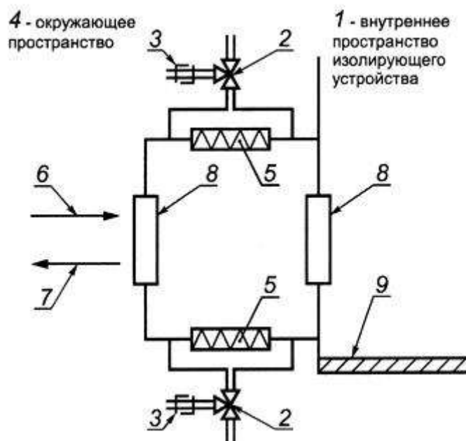
Рисунок D.8 - Передаточное устройство типа E
