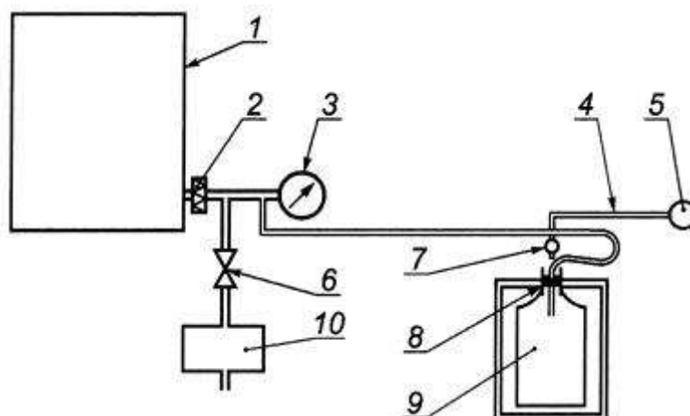
Рисунок F.3 - Типовая схема установки контрольного оборудования с его расположением вне изолирующего устройства
