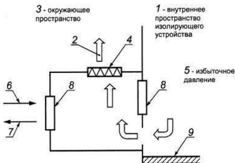
Рисунок D.5 - Передаточное устройство типа С1
