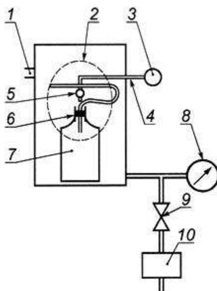
Рисунок F.2 - Типовая схема установки контрольного оборудования
