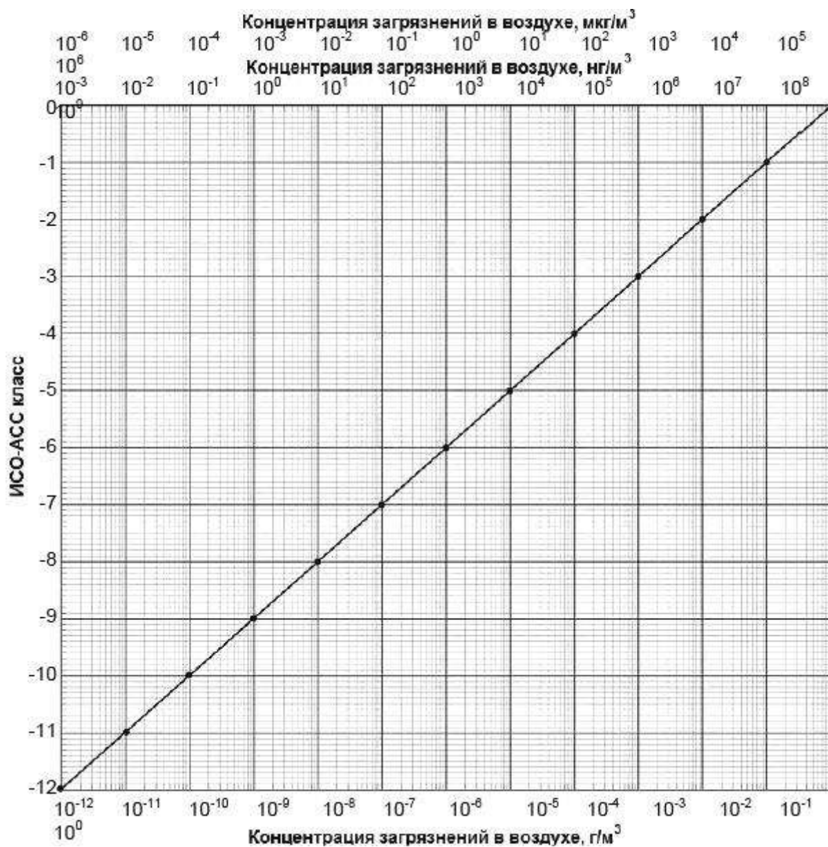
Рисунок 1 - Классы ИСО-АСС в зависимости от концентрации загрязнений
