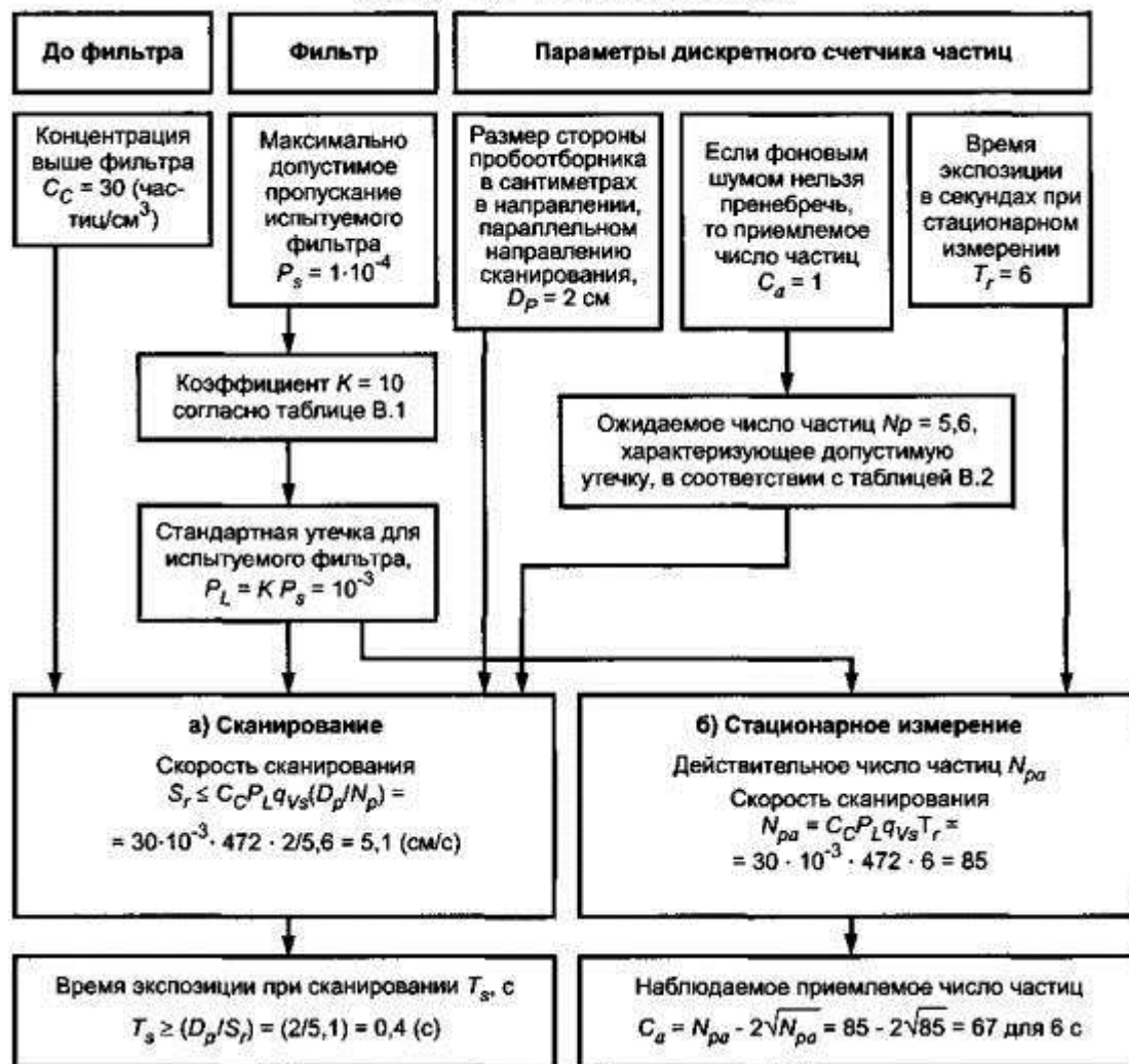
Рисунок В.3 - Схема проведения предварительных расчетов
